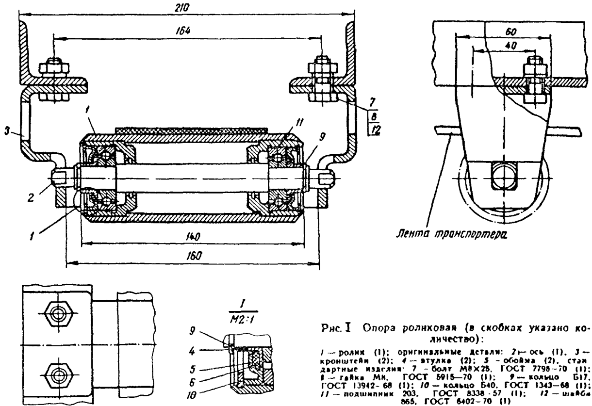
Рис. 1 Опора роликовая (в скобках указано количество):
