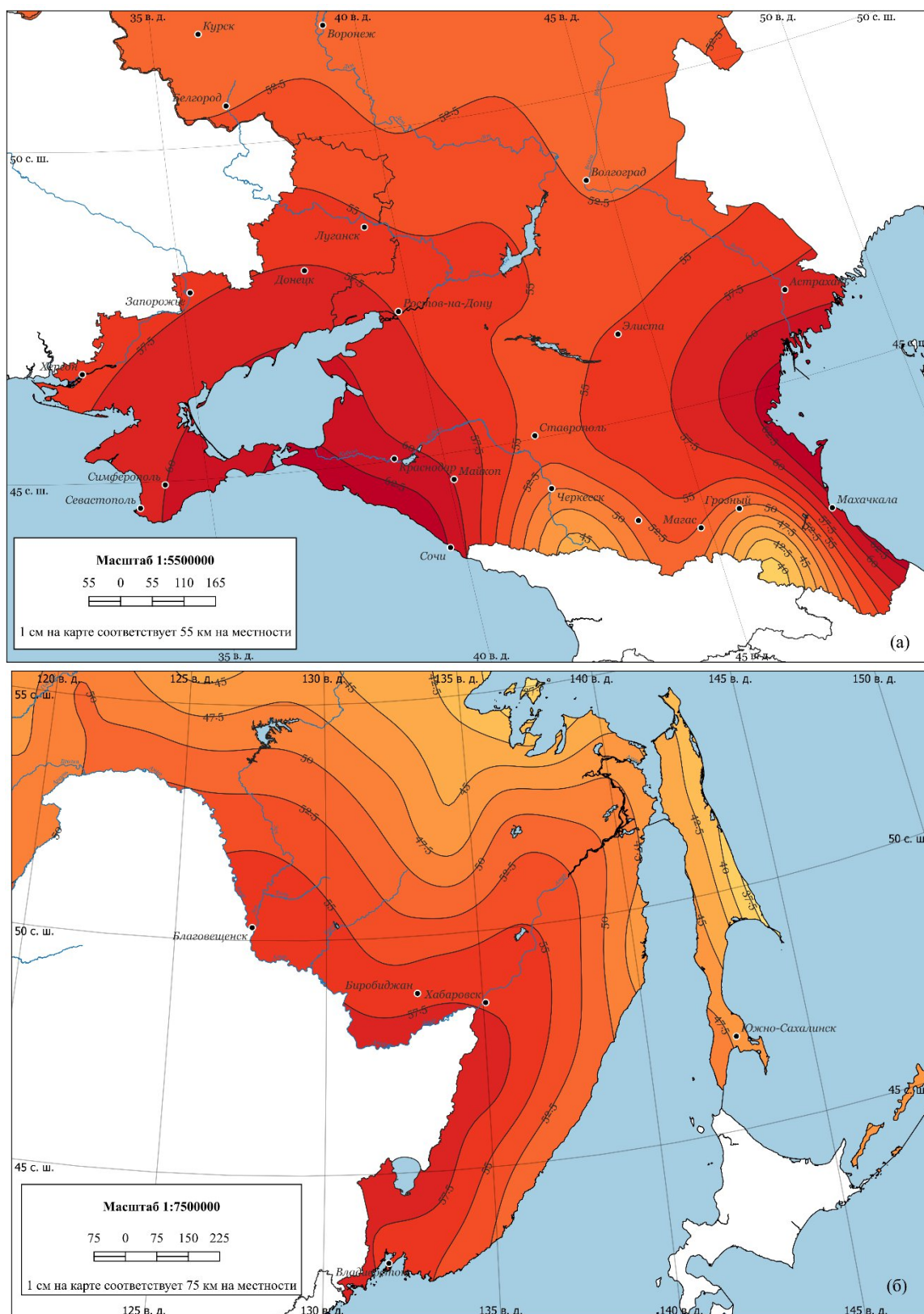
Рисунок А.7 – Схематическая карта районирования по величине удельной энтальпии I с обеспеченностью 0,95, кДж/кг, (параметр А) Южного федерального округа и территории Дальнего Востока
