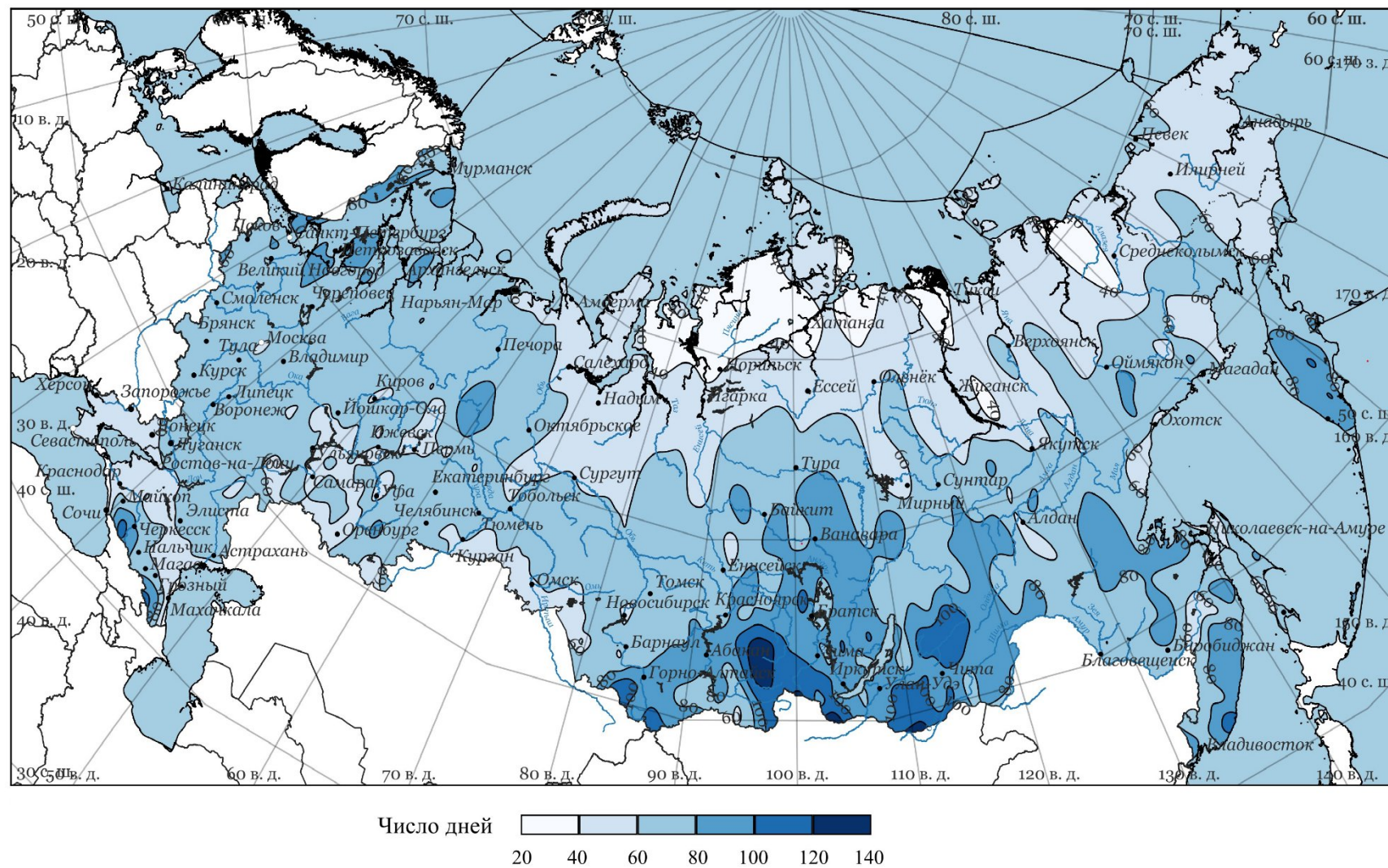
Рисунок А.3 – Схематическая карта распределения среднего за год числа дней с переходом температуры воздуха через 0 °C
