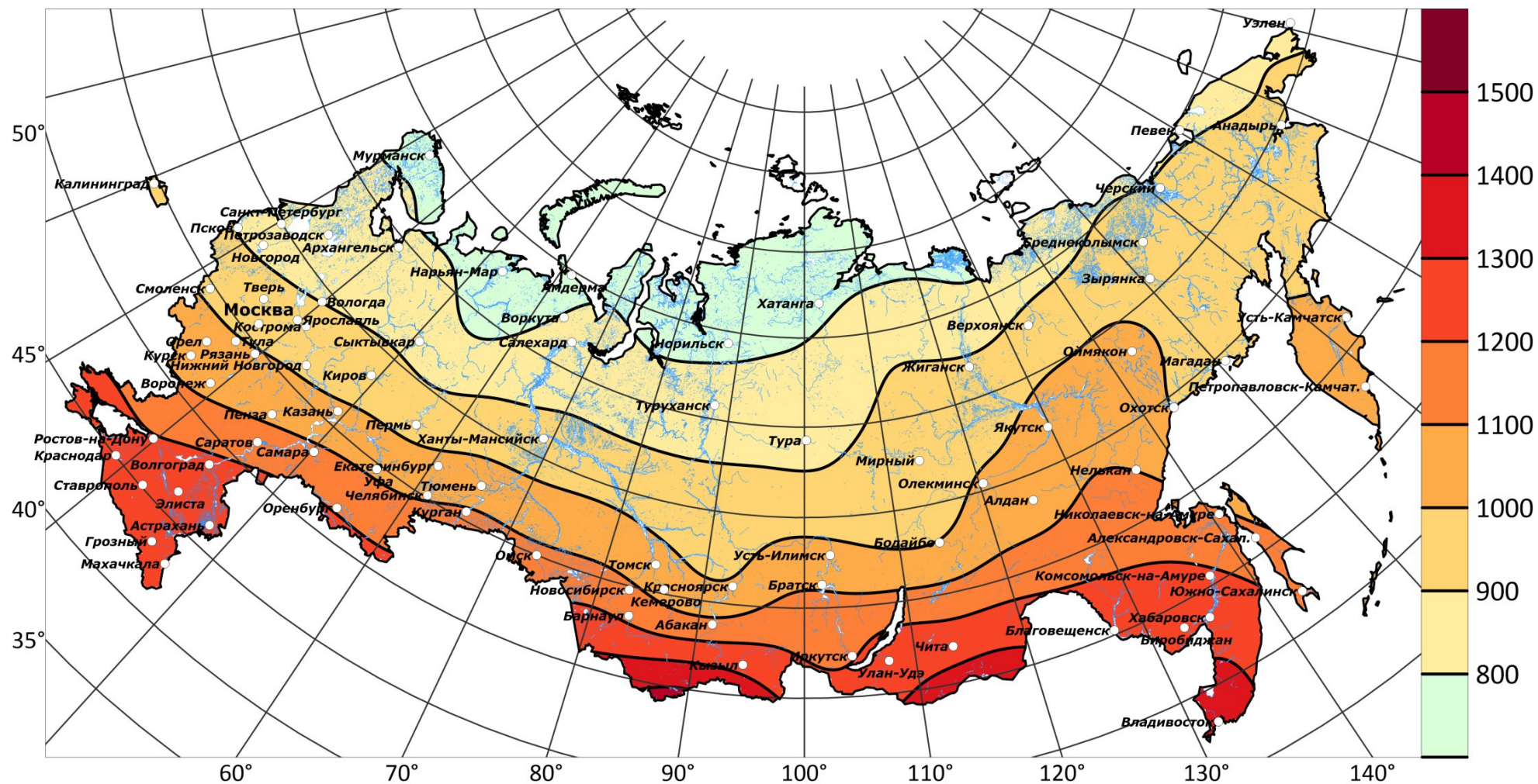
Рисунок А.9 – Схематическая карта районирования по годовому приходу суммарной солнечной радиации, поступающей на горизонтальную поверхность, при реальных условиях облачности, кВт·ч/м²
