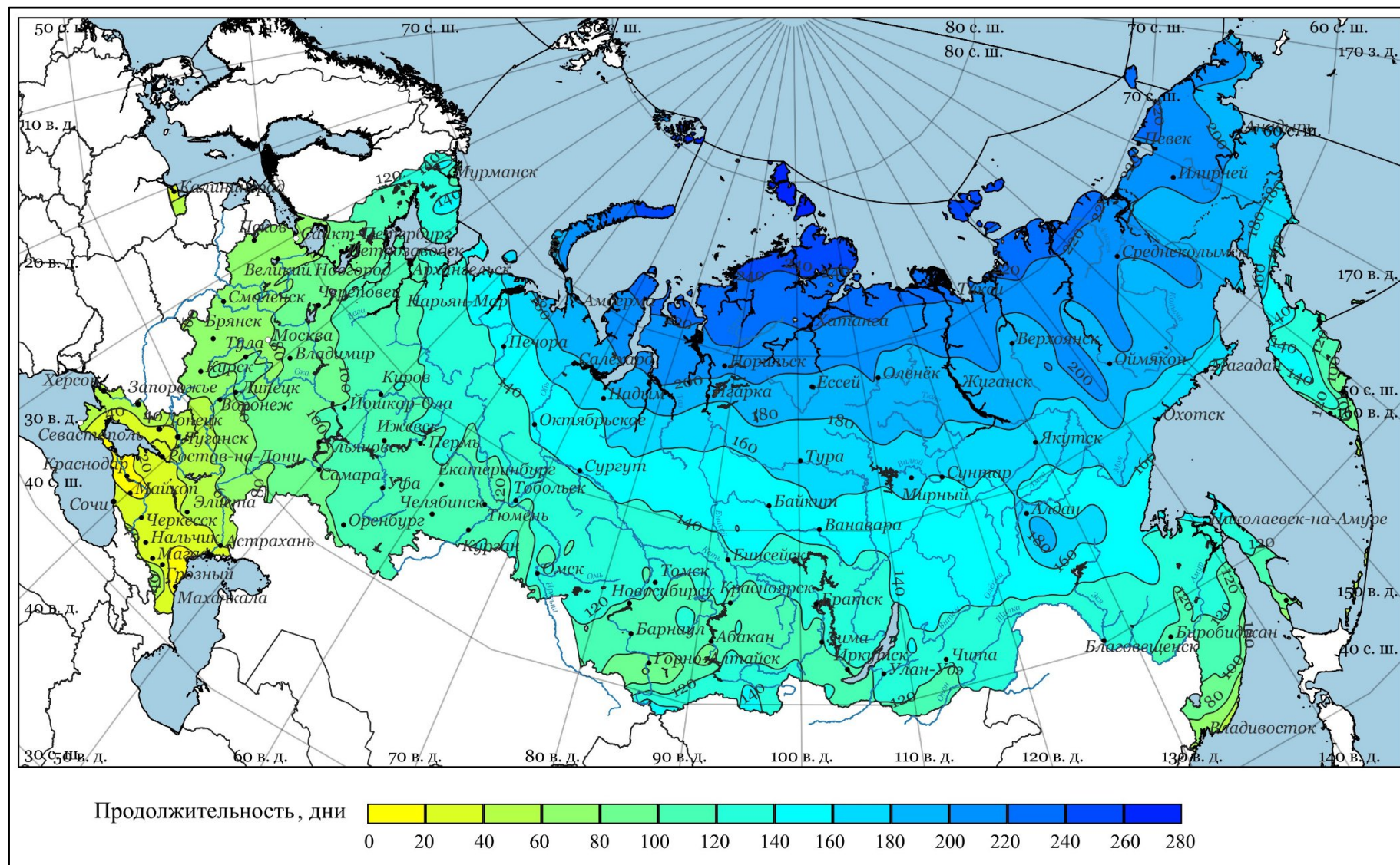
Рисунок А.10 – Схематическая карта районирования по продолжительности периода с устойчивыми морозами, дни
