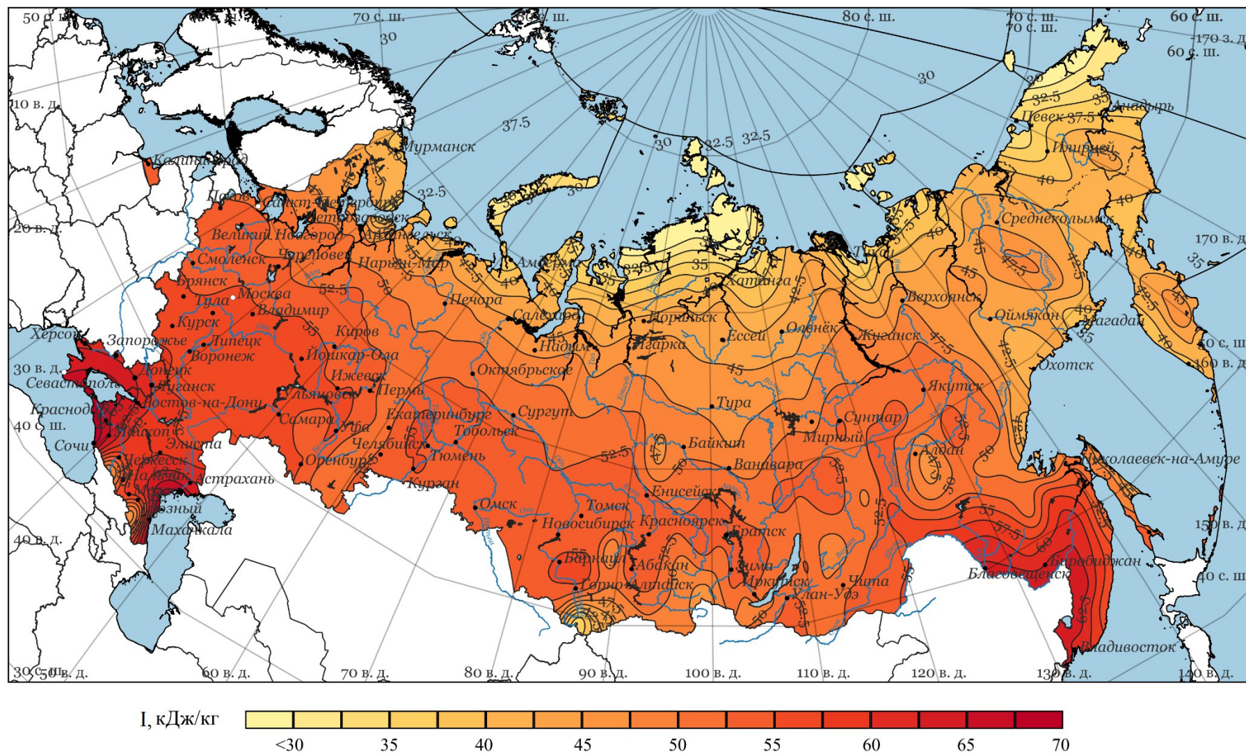
Рисунок А.6 – Схематическая карта районирования по величине удельной энтальпии I с обеспеченностью 0,98, кДж/кг (параметр Б)
