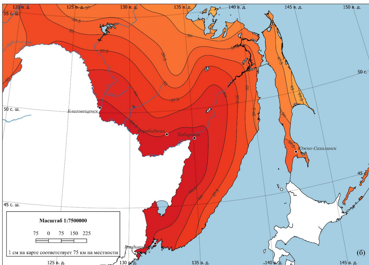
Рисунок А.8 – Схематическая карта районирования по величине удельной энтальпии I с обеспеченностью 0,98, кДж/кг, (параметр Б) Южного федерального округа и территории Дальнего Востока
