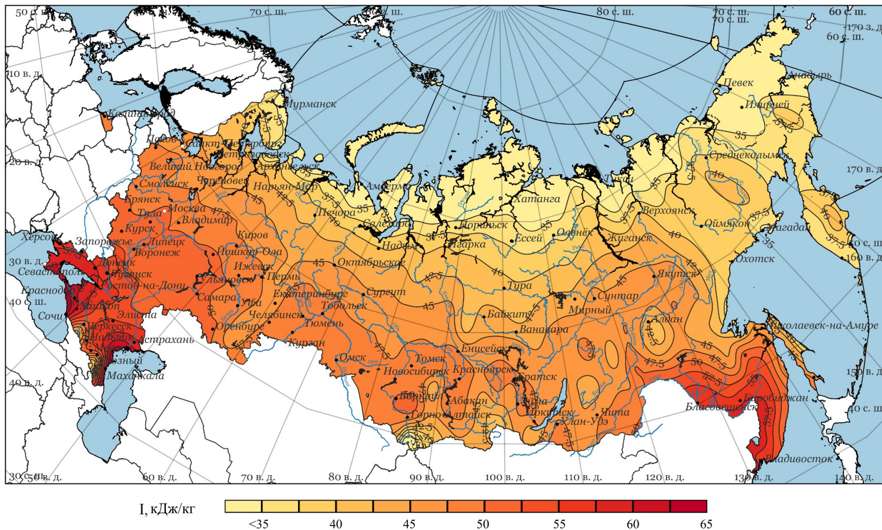
Рисунок А.5 – Схематическая карта районирования по величине удельной энтальпии I с обеспеченностью 0,95, кДж/кг (параметр А)
