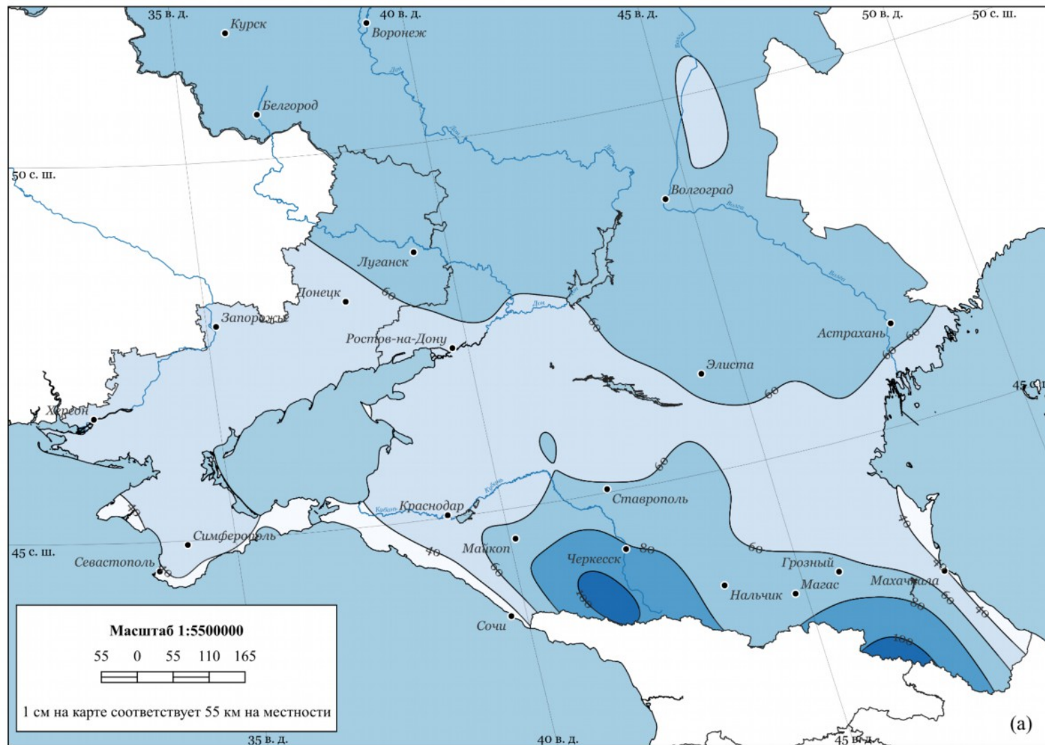
Рисунок А.4 – Схематическая карта распределения среднего за год числа дней с переходом температуры воздуха через 0 °С Южного федерального округа
