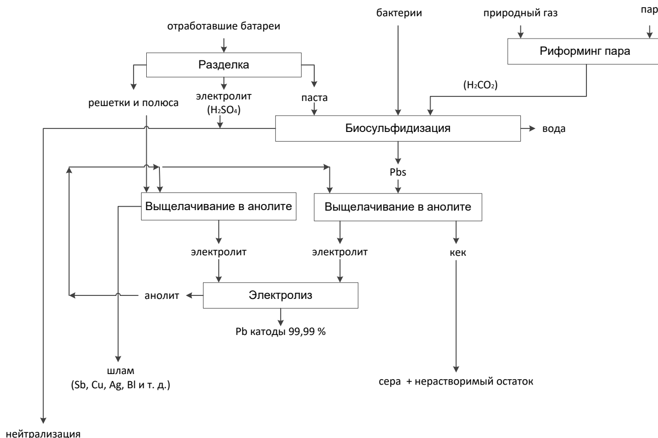
Рисунок 2.26 — Принципиальная схема THIOPAQ® + FLUBOR®-процесса
