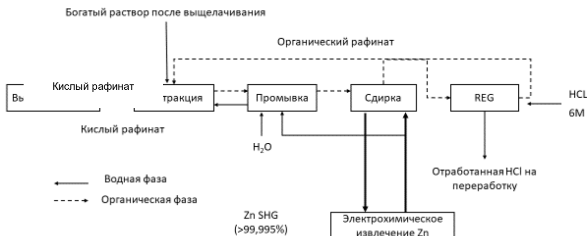
Рисунок 2.8 — Упрощенная схема модифицированного процесса Zincex™ (экстракция растворителем)
