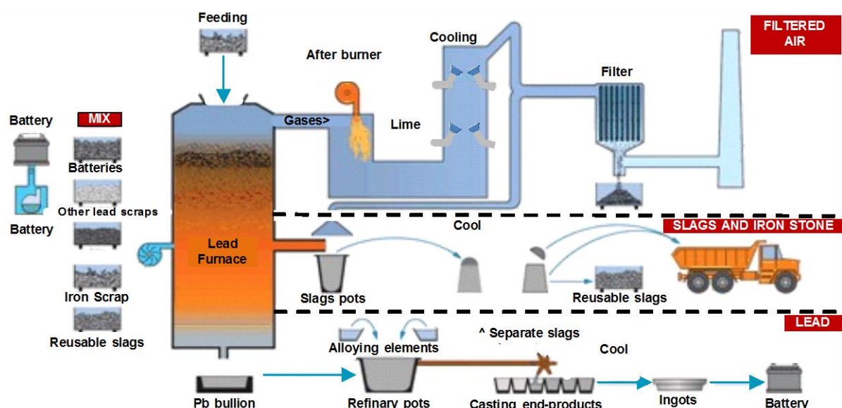
Рисунок 2.19 — Схема типичного процесса восстановления аккумуляторных батарей в шахтной печи
