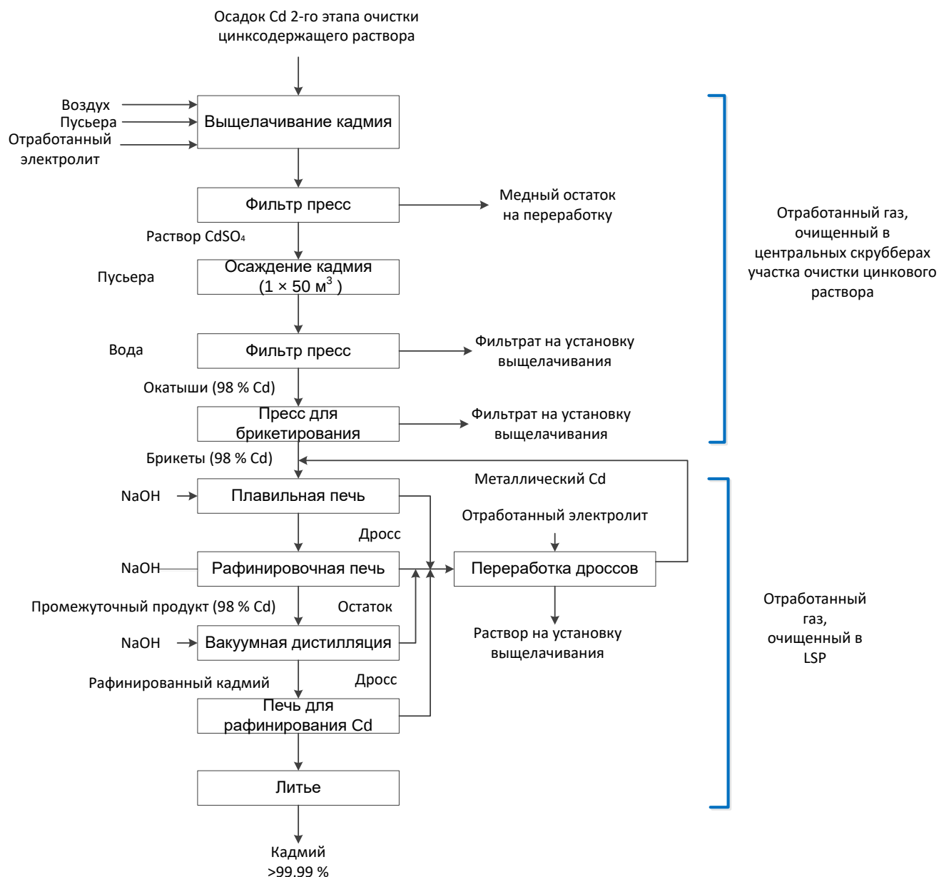
Рисунок 2.15 — Схема процесса производства кадмия: завод F
