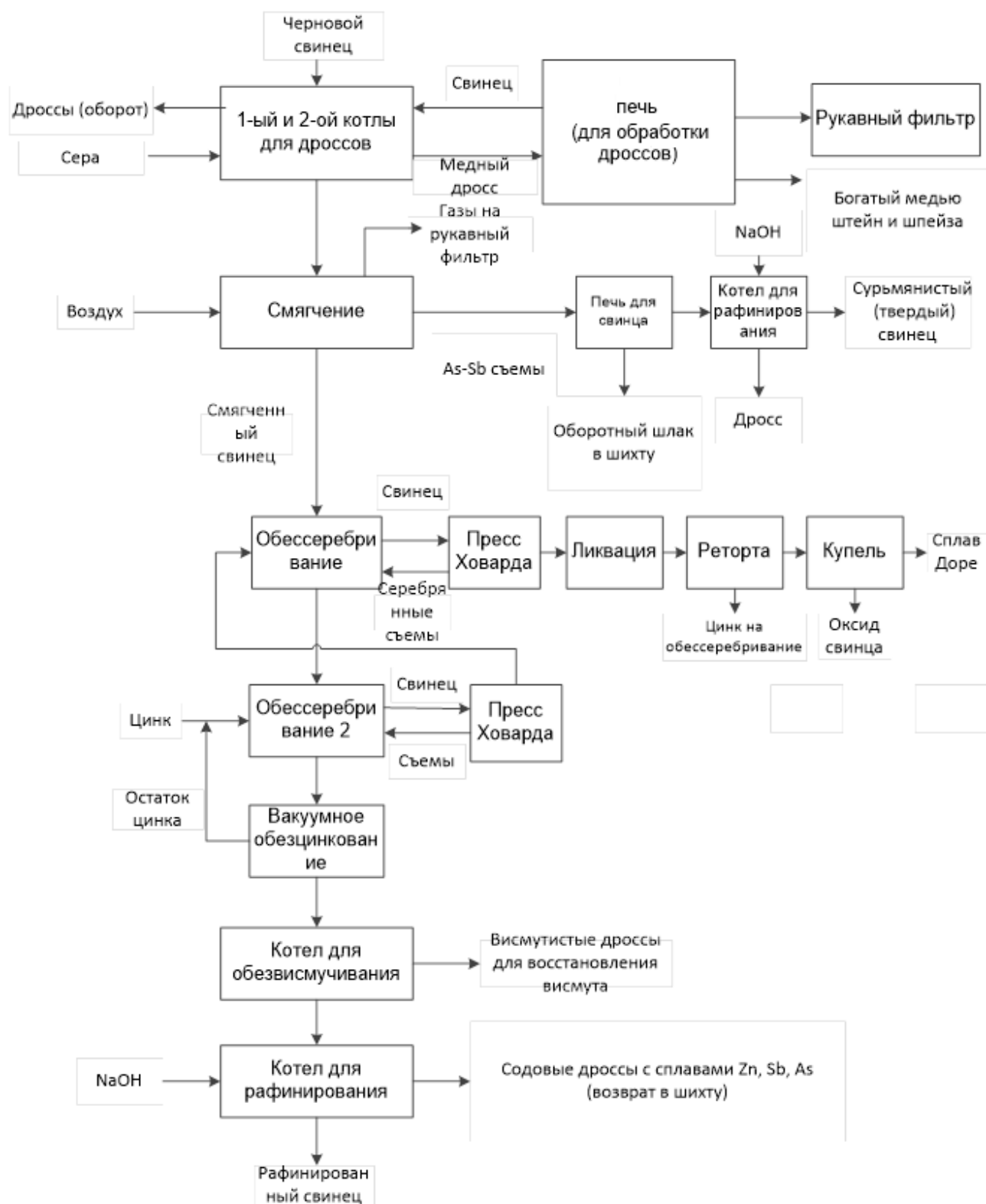
Рисунок 2.27 — Примерная схема процессов рафинирования свинца
