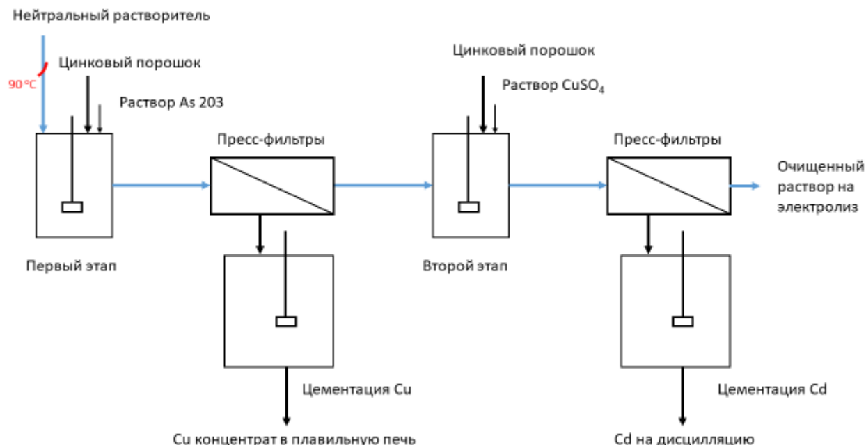
Рисунок 2.6 — Пример схемы процесса очистки, основанного на As, для удаления Co и Ni
