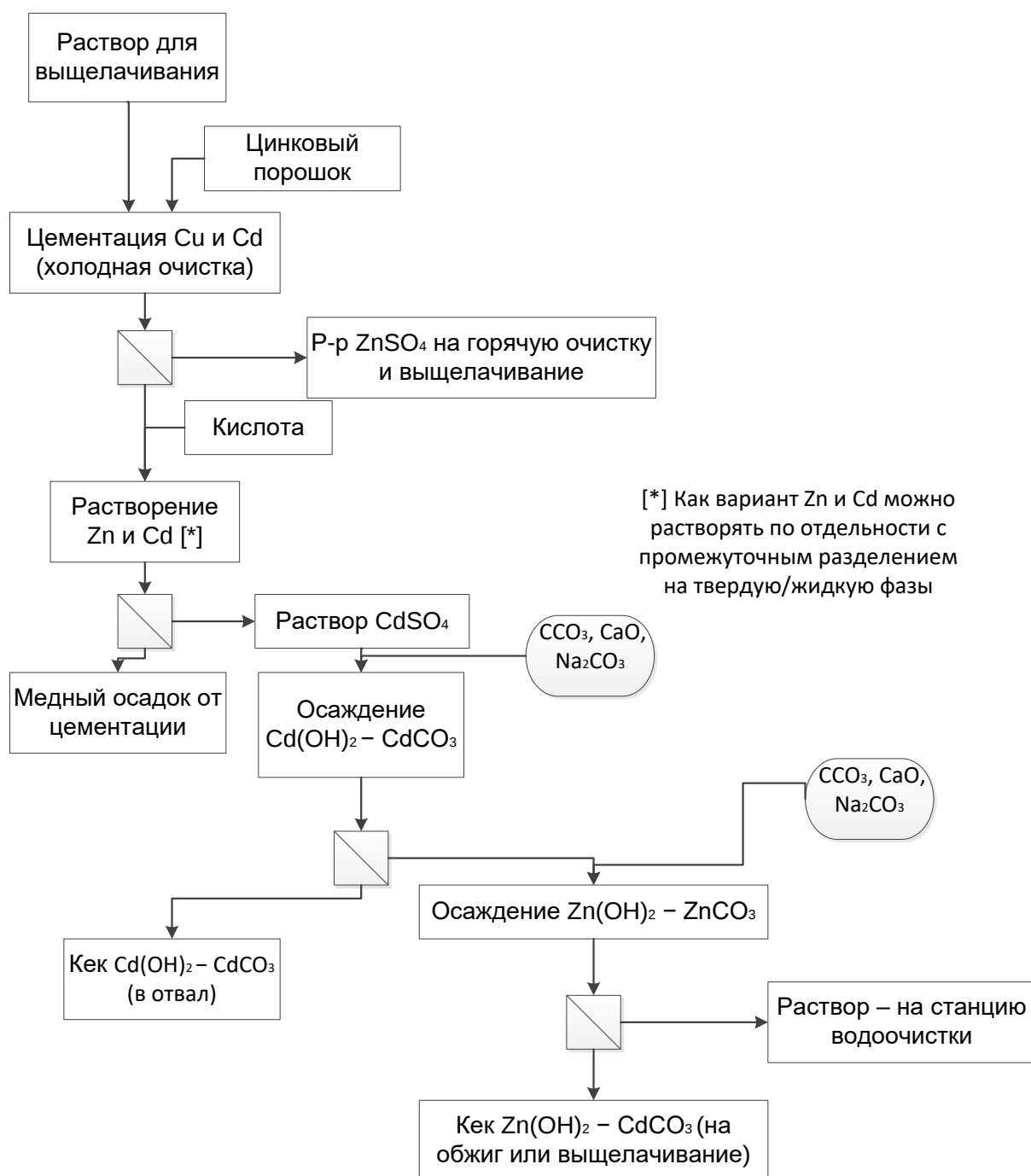
Рисунок 2.14 — Схема процесса производства кадмия: завод Е
