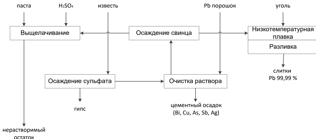
Рисунок 2.24 — Принципиальная схема PLINT-процесса
