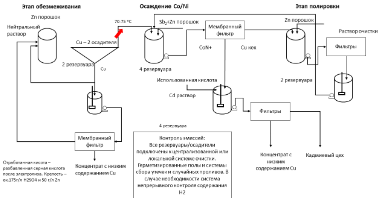
Рисунок 2.7 — Схема процесса очистки на основе сурьмы на одном из европейских заводов
