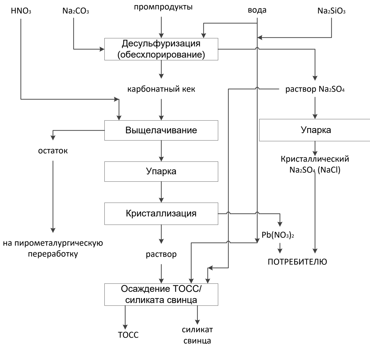
Рисунок 2.21 — Принципиальная технологическая схема получения химических соединений свинца из промпродуктов переработки батарей (трехосновный сульфат свинца (ТОСС))
