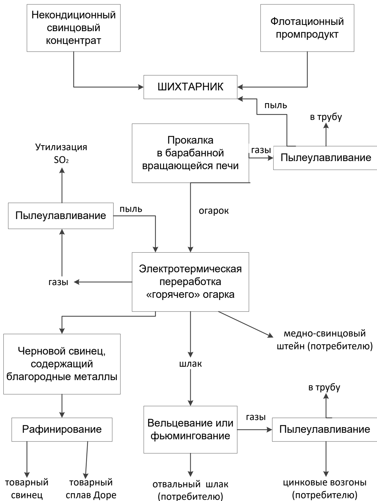
Рисунок 6.6 — Технологическая схема безотходной переработки некондиционных концентратов, содержащих благородные металлы
