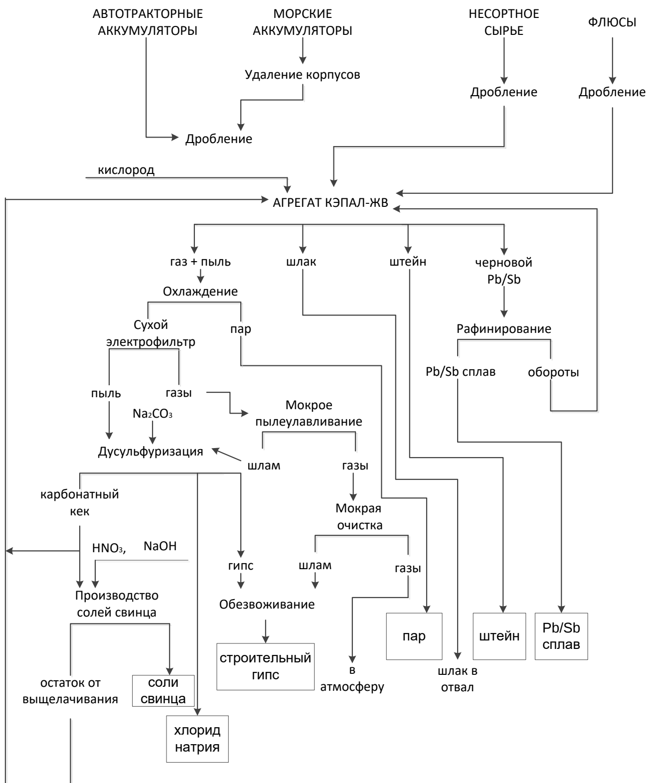
Рисунок 6.4 — Технологическая схема переработки лома свинцовых аккумуляторов без предварительной разделки
