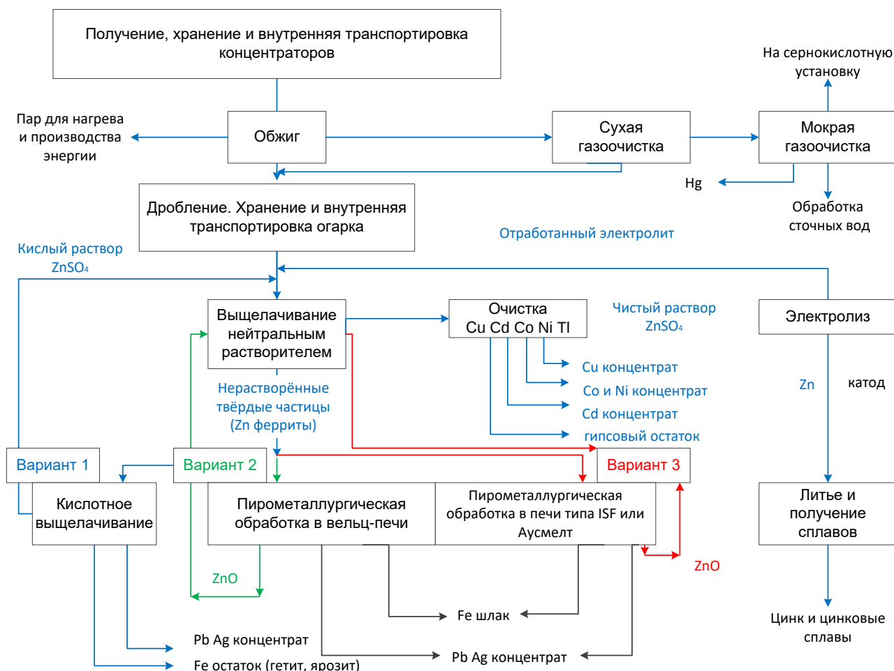
Рисунок 2.1 — Упрощенная схема гидрометаллургического способа
