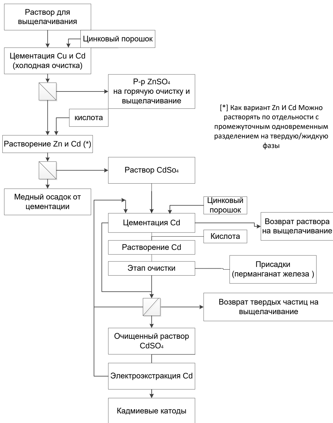
Рисунок 2.11 — Схема процесса производства кадмия: завод В
