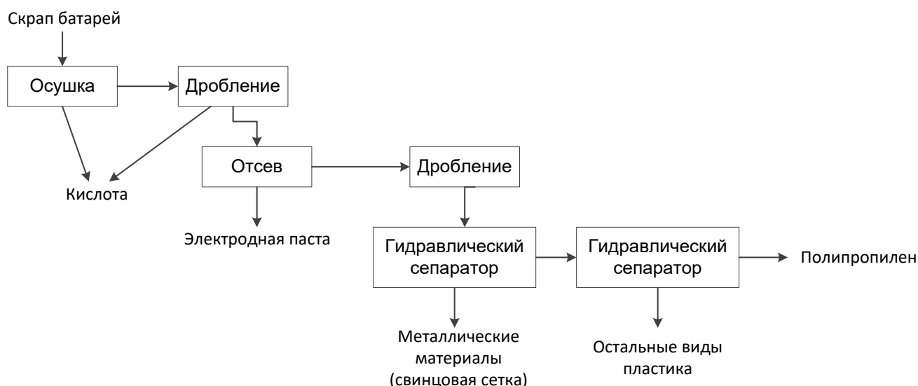
Рисунок 2.18 — Схема типового процесса переработки аккумуляторных батарей
