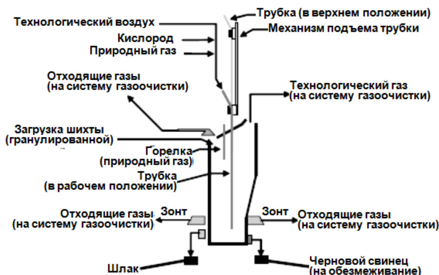
Рисунок 2.16 — Схема печи Ausmelt
