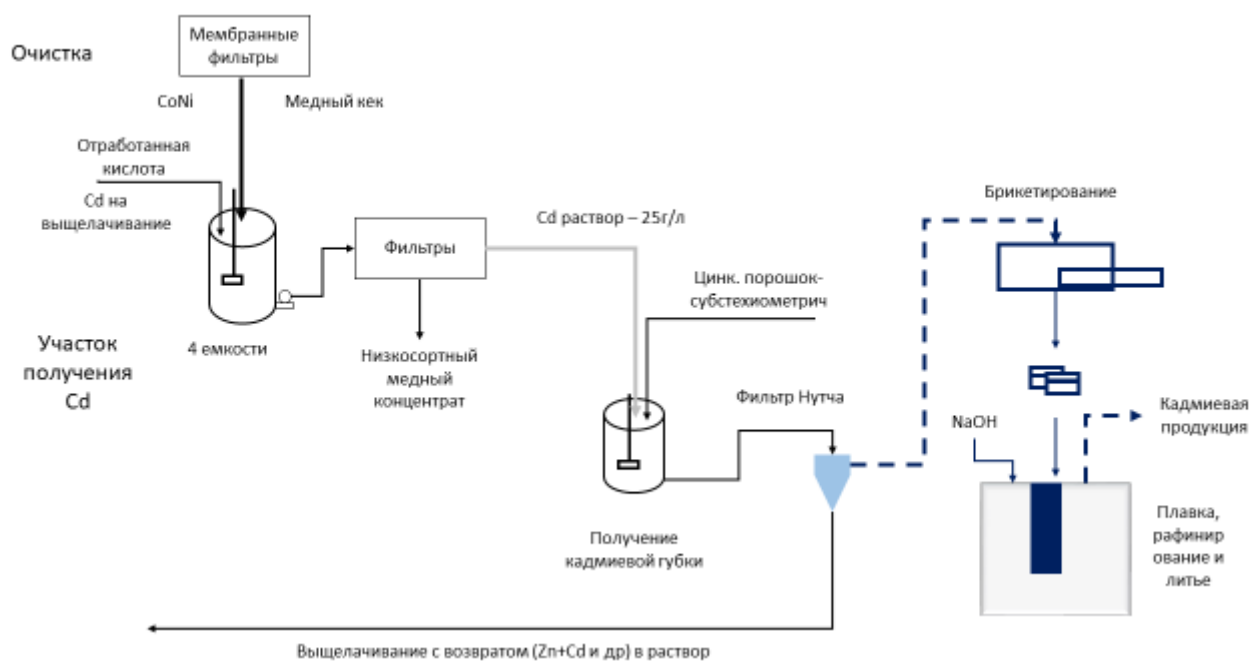
Рисунок 2.13 — Схема процесса производства кадмия: завод D
