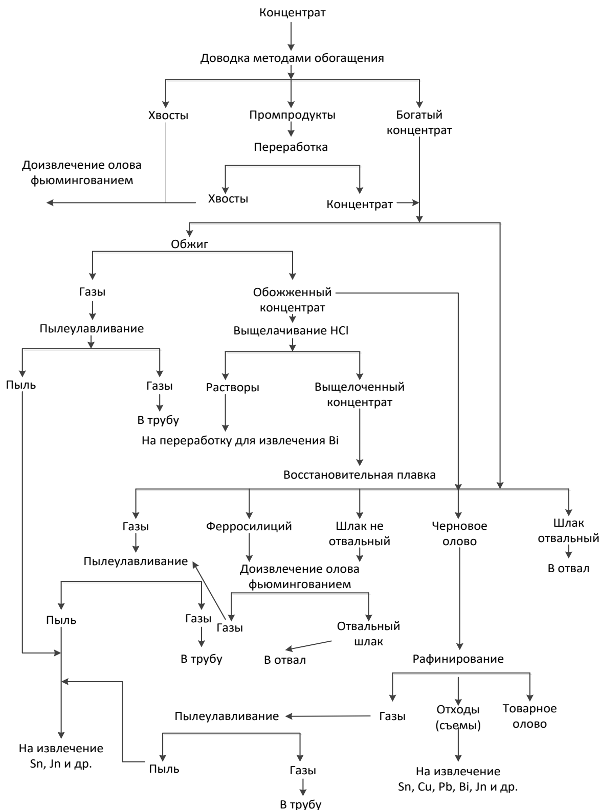
Рисунок 2.17 — Принципиальная технологическая схема переработки оловянных концентратов на товарное олово
