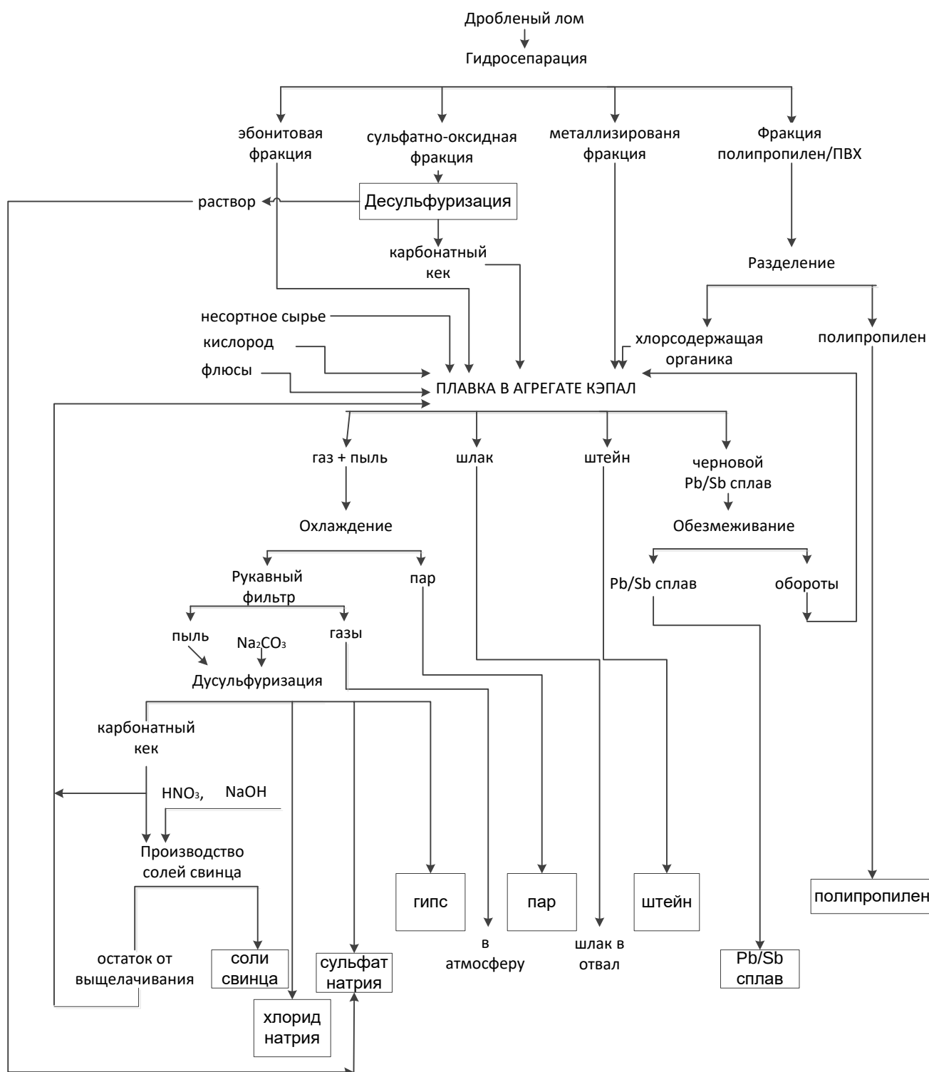
Рисунок 6.5 — Технологическая схема переработки лома свинцовых аккумуляторов с предварительной разделкой
