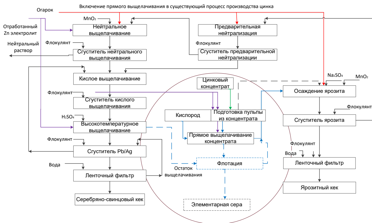
Рисунок 2.5 — Схема процесса выщелачивания с применением прямого выщелачивания при атмосферном давлении для повышения мощности завода
