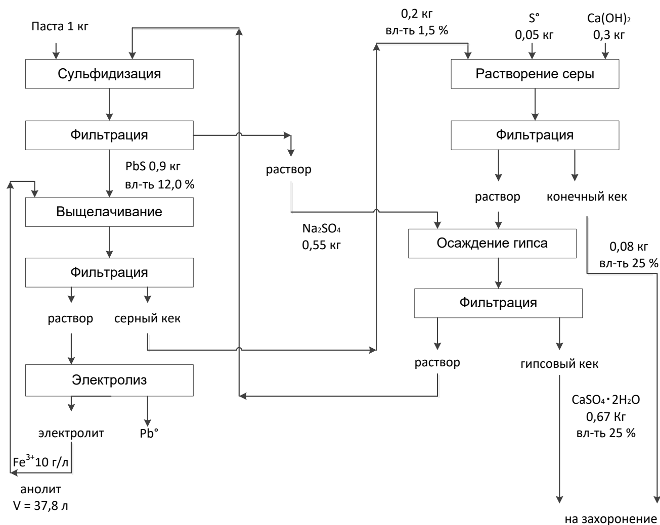
Рисунок 2.25 — Принципиальная схема CX-EWS + FLUBOR®-процесса
