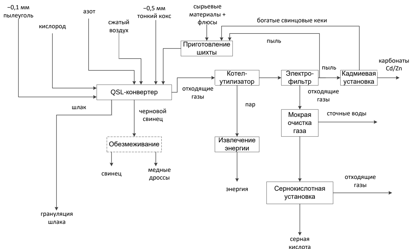
Рисунок 6.1 — Схема QSL-завода в Штольберге (Германия)
