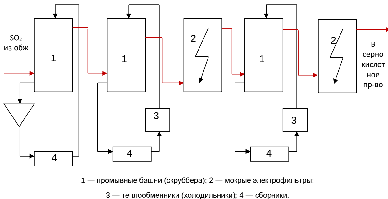
Рисунок 2.3 — Второй этап очистки отходящего газа обжиговой печи: мокрая очистка газа
