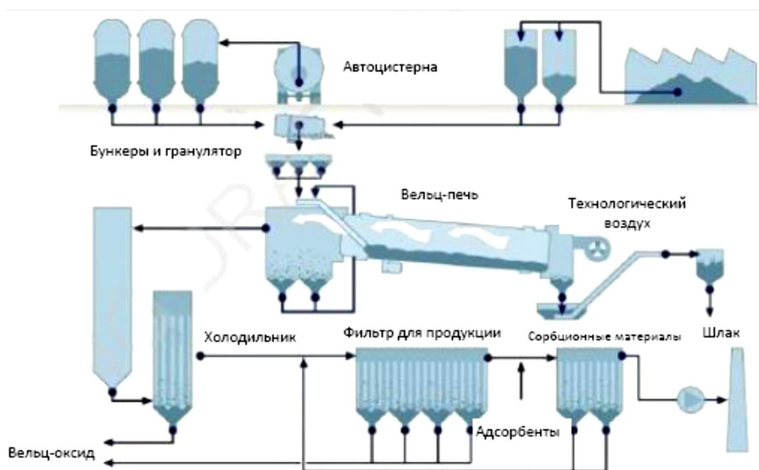
Рисунок 2.9 — Технологическая схема вельц-процесса
