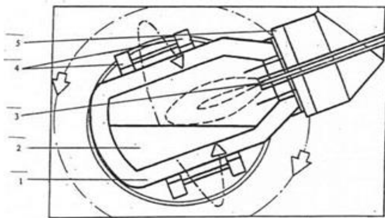
1 — кожух конвертера; 2 — расплав; 3 — фурма; 4 — опорно-поворотное устройство; 5 — напыльник, содержащий \text{SO}_2 . Газы направляются на сернокислотный завод после обеспыливания и сушки
