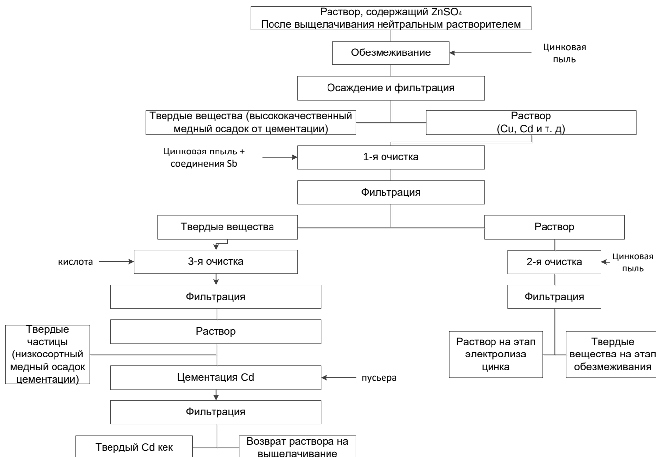
Рисунок 2.12 — Технологическая схема очистки, включая производство кадмия: завод С
