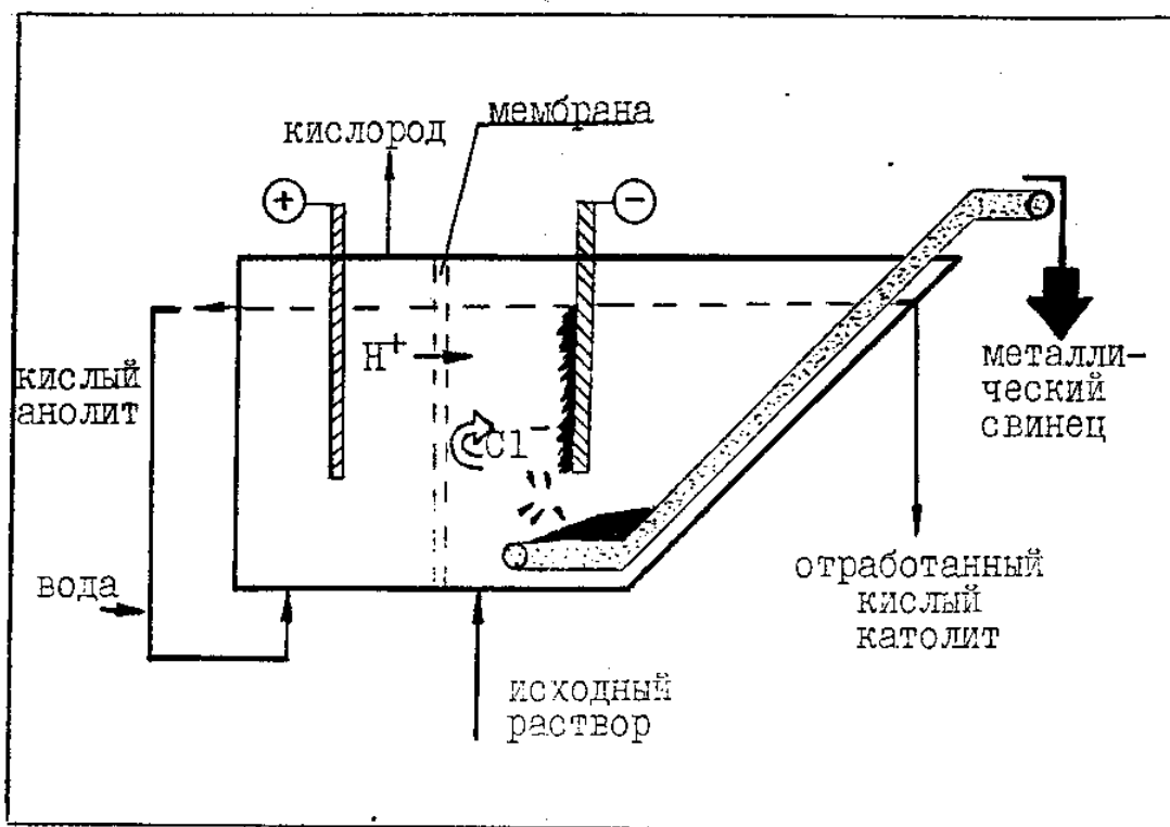
Рисунок 2.23 — Схема электроосадительной ванны PLACID
