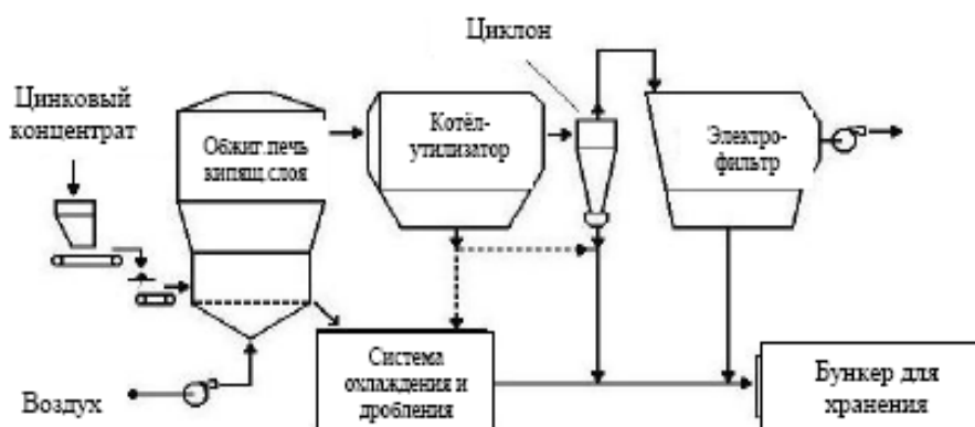
Рисунок 2.2 — Первый этап очистки отходящего газа обжиговой печи — очистка сухого газа (циклон устанавливается при необходимости)
