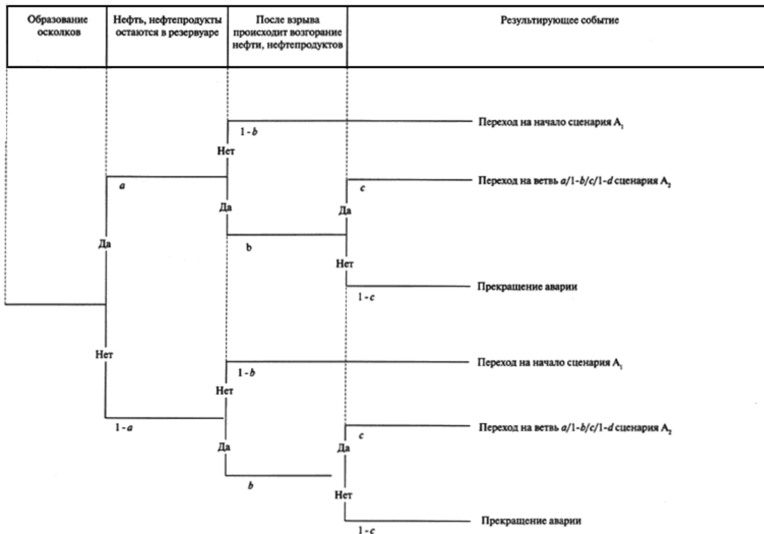
Рис.1-3. Дерево событий при взрыве внутри наземного резервуара
