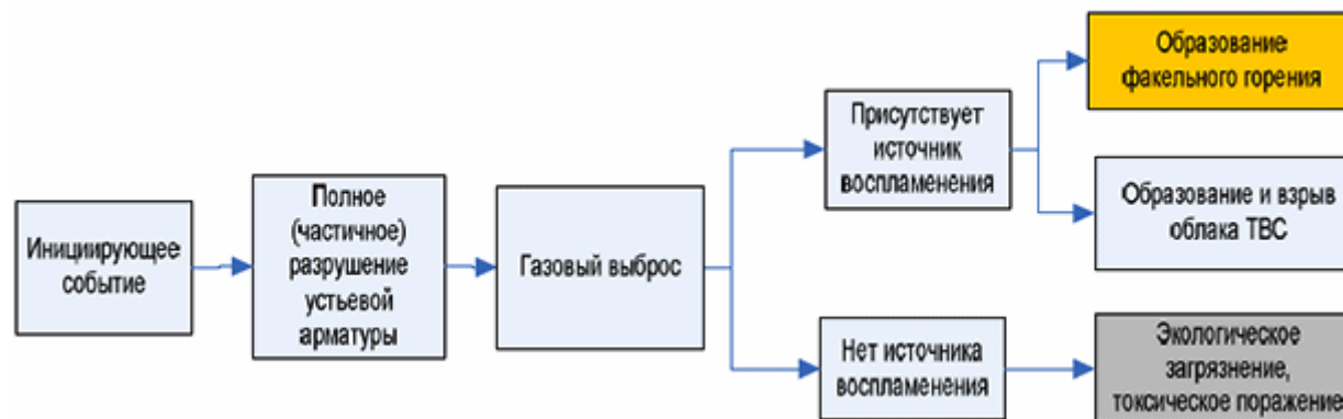
Рис.1-11. Скважины газовые
