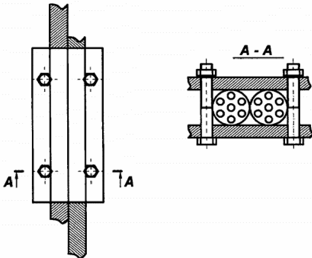
Рисунок 4. Схема соединения двух отрезков заземляющих тросов
