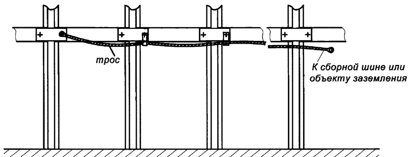
Рисунок 11. Устройства местного заземлителя с помощью рамной крепи
