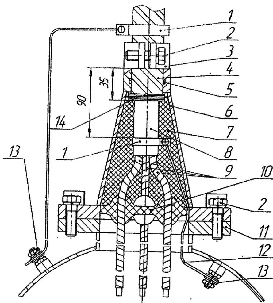
Рисунок 13. Заземление бронированного кабеля с бумажной изоляцией в вводном устройстве рудничного электрооборудования с заливкой кабельной мастикой: 1 - заземляющий хомут с зажимом; 2 - болты; 3 - зажим; 4 - стальная броня; 5 - кольцо уплотнительное; 6 - муфта; 7 - мастика; 8 - свинцовая оболочка; 9 - изоляция жилы;
