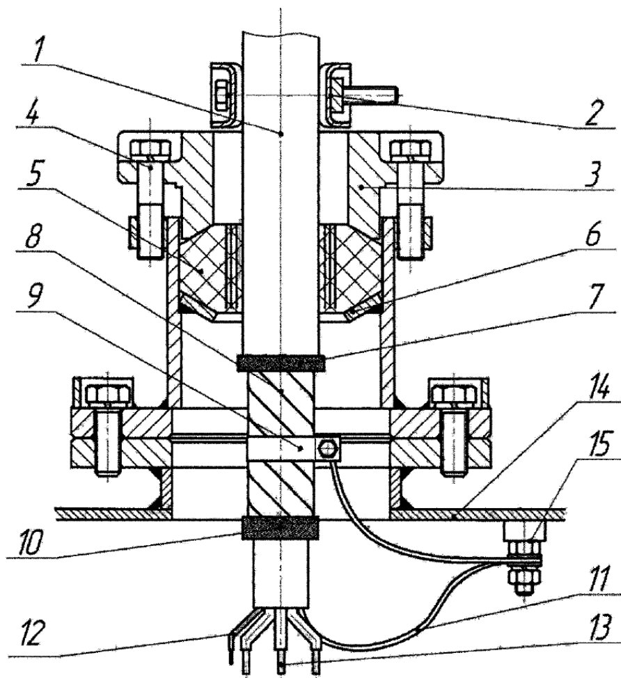
Рисунок 14. Заземление бронированного кабеля с пластмассовой изоляцией во вводном устройстве рудничного электрооборудования: 1 - кабель; 2 - нажимная скоба; 3 - муфта; 4 - болт; 5 - кольцо уплотнительное; 6 - гнездо; 7 и 10 - бандажи; 8 - броня; 9 - хомут на броню для заземления; 11 - жила заземления; 12 - вспомогательная жила кабеля; 13 - силовая жила; 14 - корпус вводной камеры; 15 - внутренний зажим заземления
