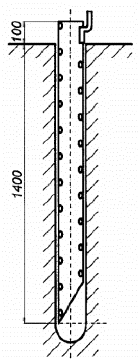
Рисунок 8. Схема расположения заземлителя в шпуре
