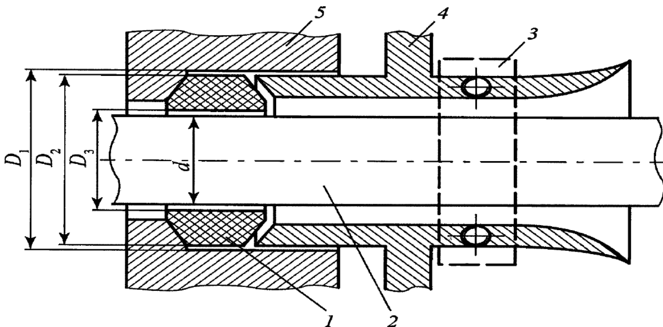
Рисунок. Схема расположения элементов во вводном устройстве до момента сжатия уплотнительного кольца: 1 - уплотнительное кольцо; 2 - кабель; 3 - закрепляющая планка; 4 - уплотняющий фланец; 5 - корпус оболочки
