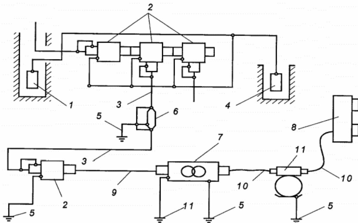
Рисунок 1. Схема общего заземляющего устройства шахты:
