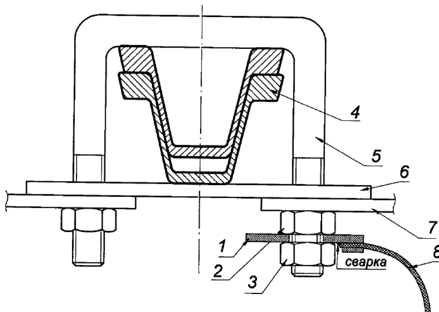
Рисунок 10. Пример присоединения заземляющего проводника к металлической рамной креплё: 1 - стальной наконечник; 2 - гайка; 3 - дополнительная гайка; 4 - специальный взаимозаменяемый профиль (СВП); 5 - скоба; 6 - планка; 7 - межрамная стяжка; 8 - заземляющий проводник
